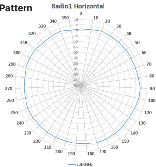
H-Plane Pattern
